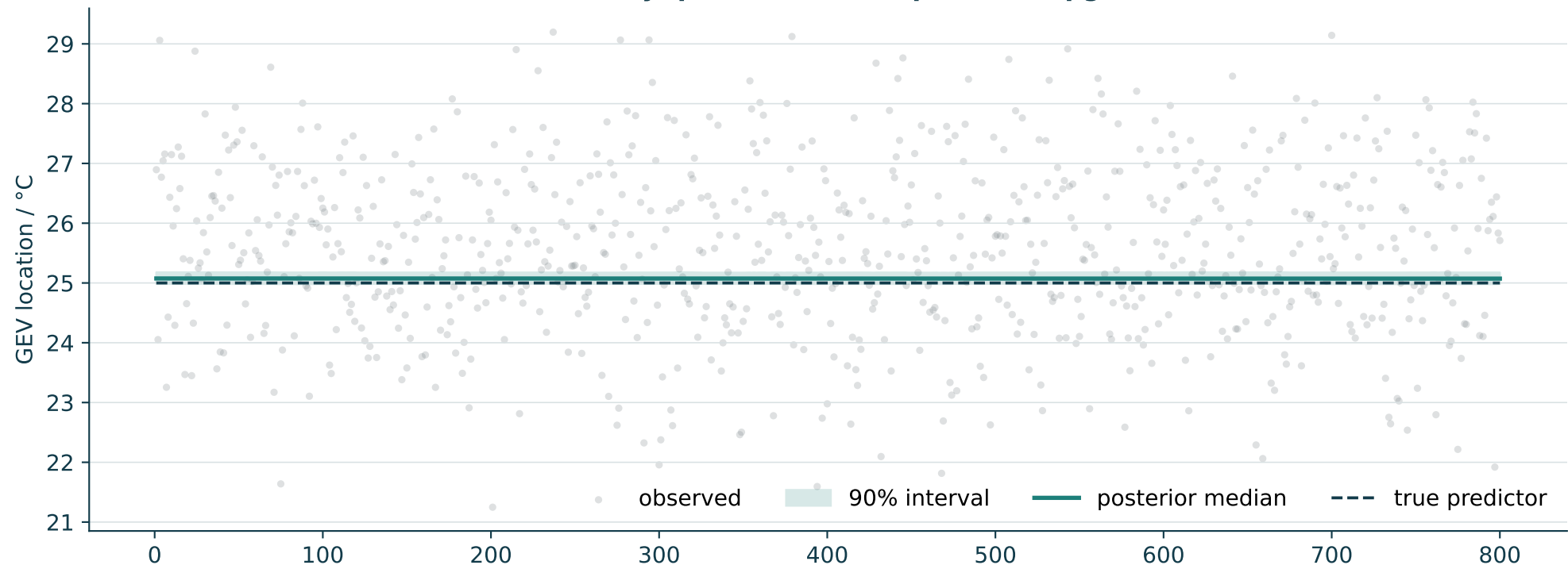
stationary: posterior latent predictor (pgas)
