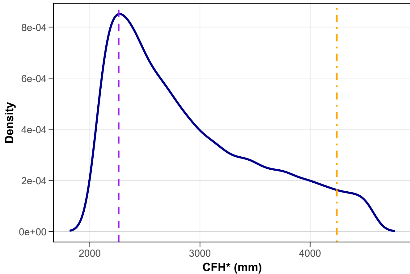
CFH* posterior ( \xi prior: improper)
