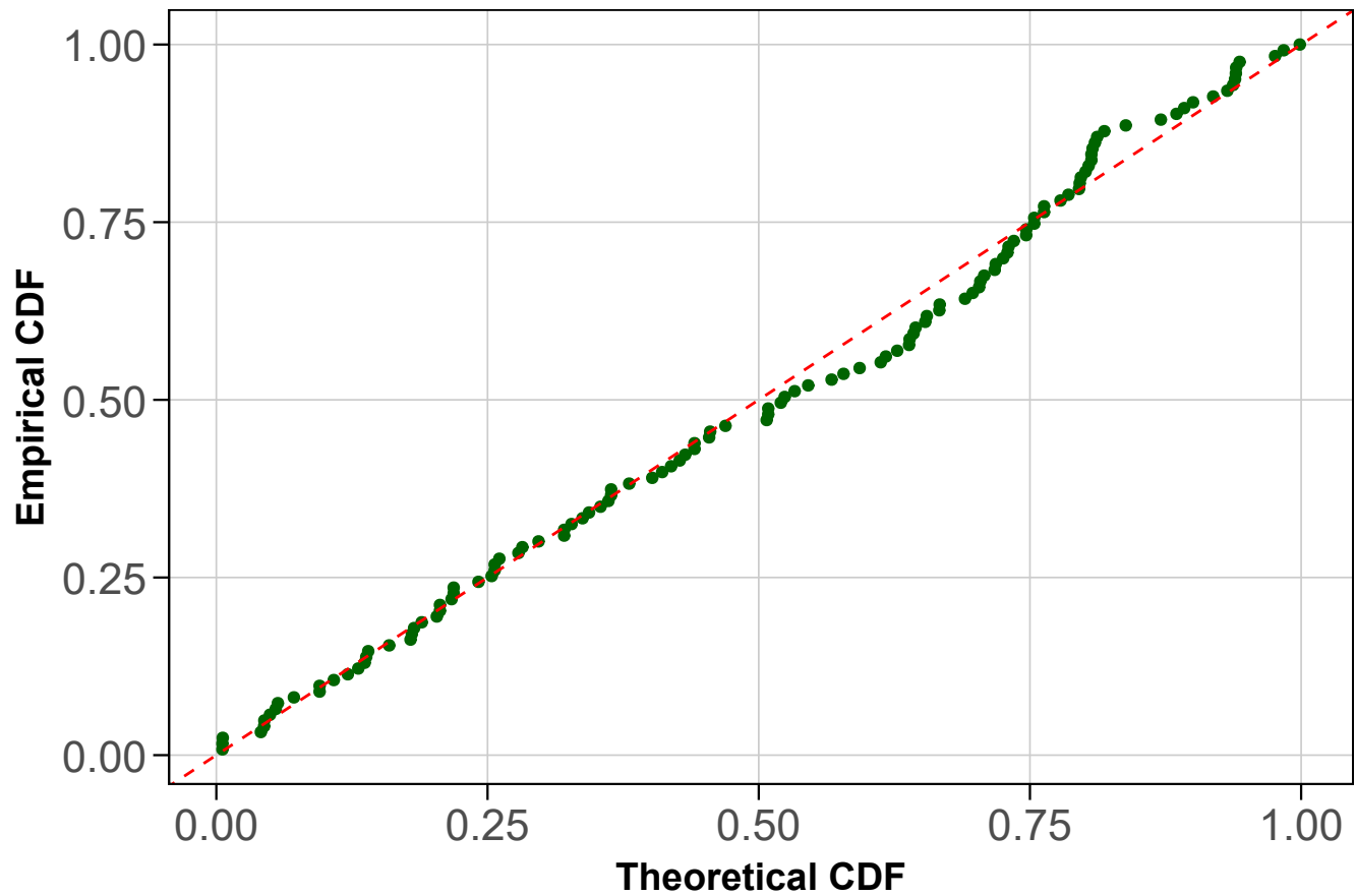
P-P plot: GPD
