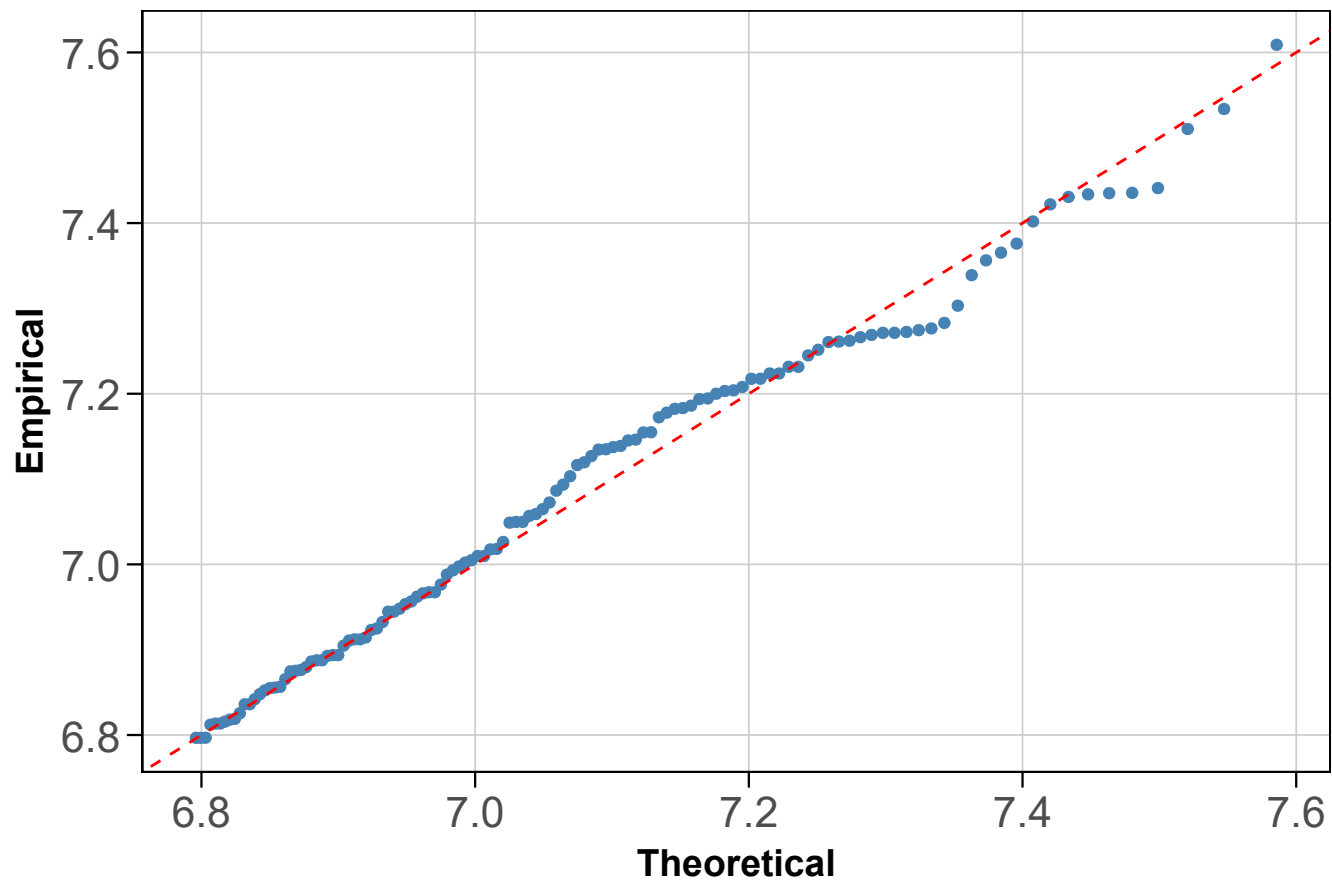
Q-Q plot: GPD
