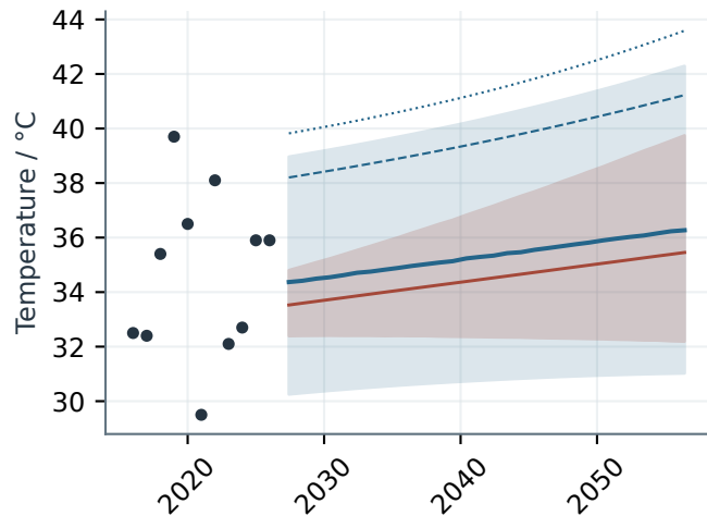
TXx &gt; 39.7 °C
