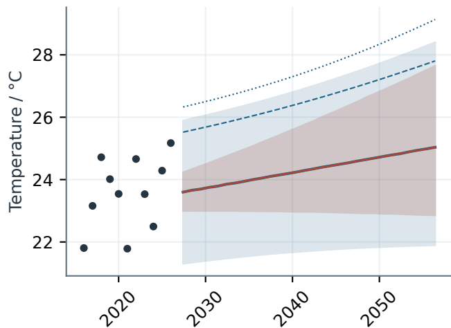
TXx &gt; 35 °C
