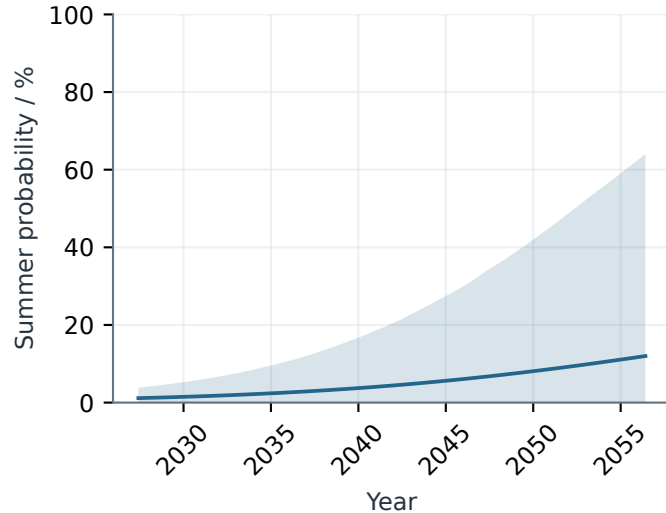
TXx &gt; 39.7 °C
