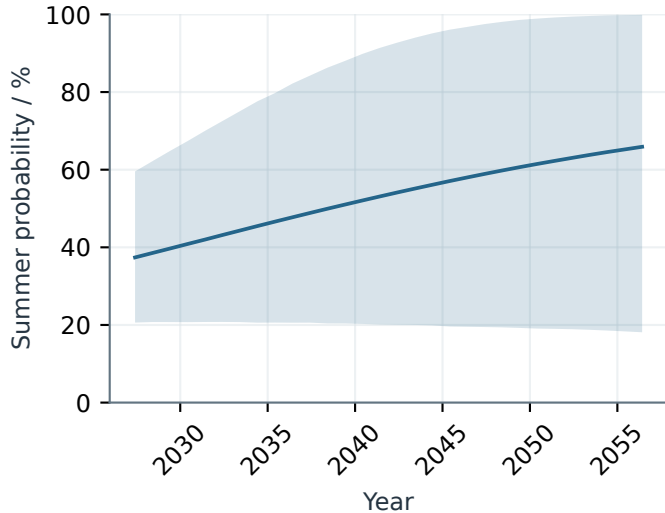
TXx &gt; 35 °C
