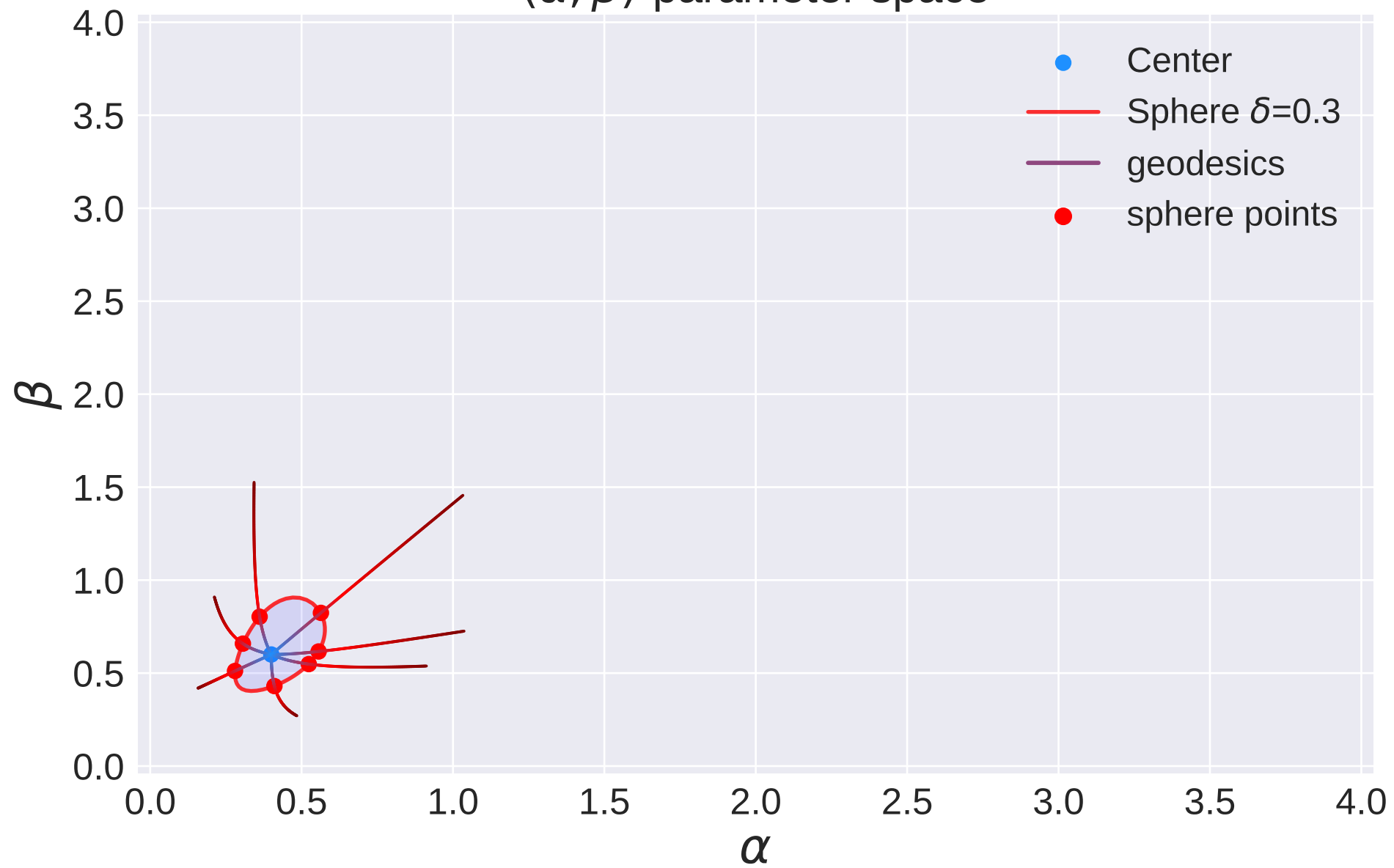
(\alpha, \beta) -parameter space
