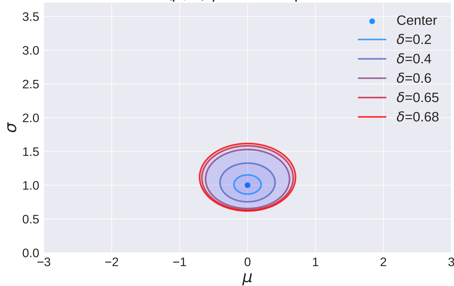
(\mu, \sigma) -parameter space
