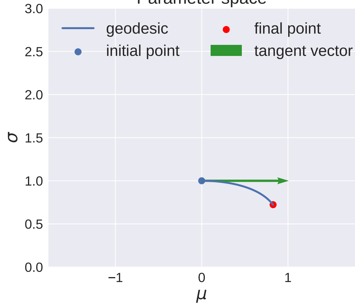
Parameter space
