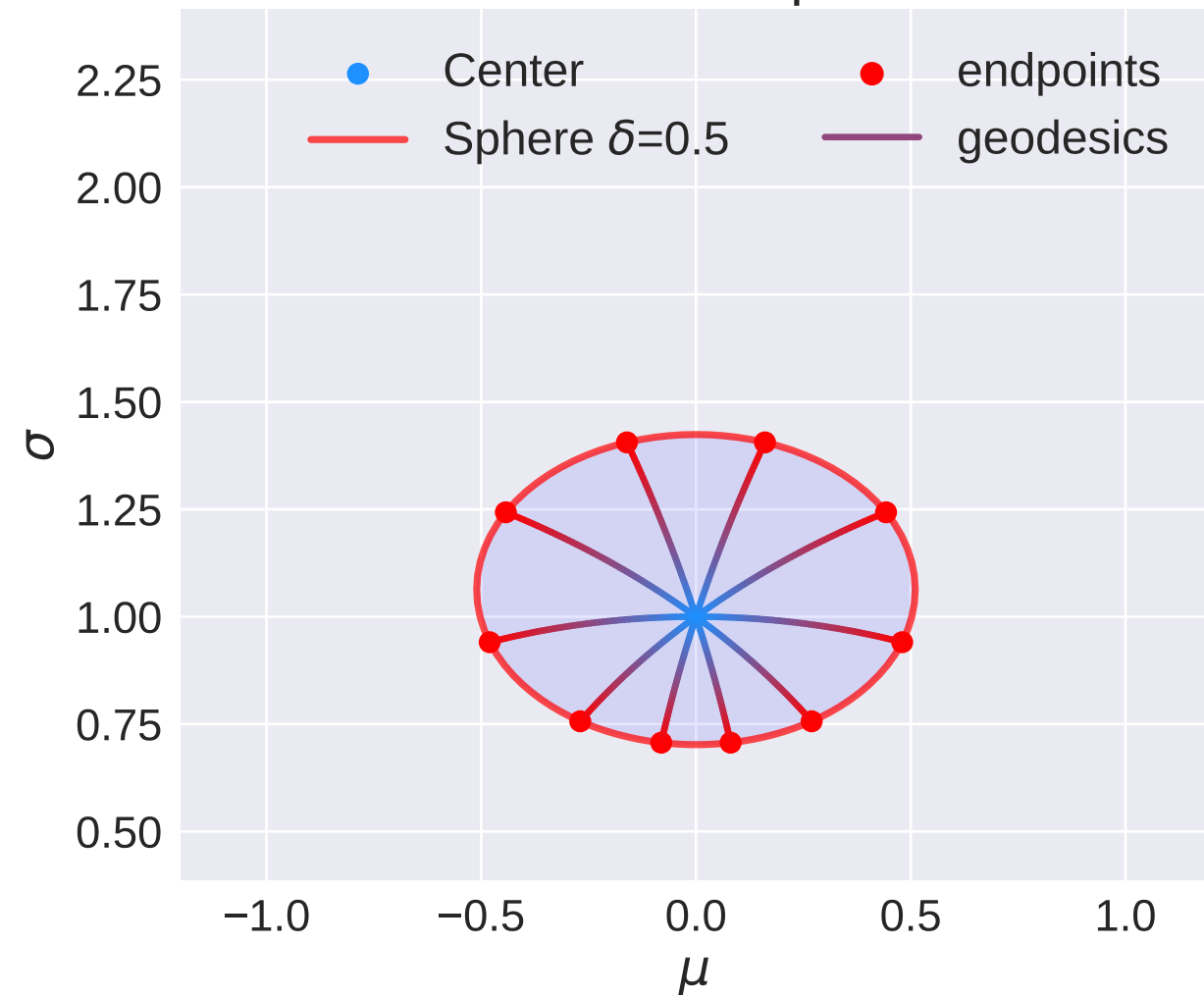
Parameter space
