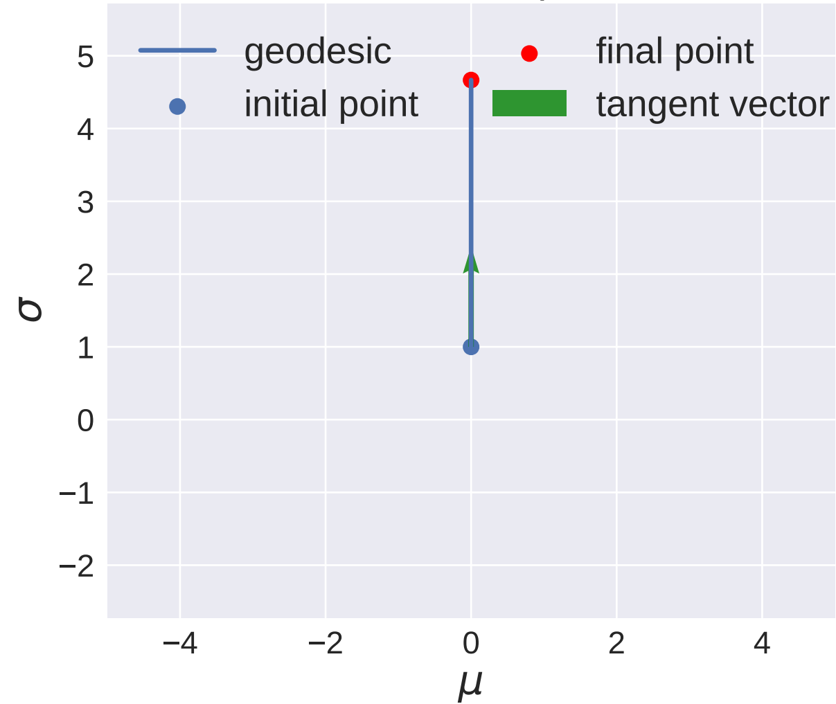
Parameter space
