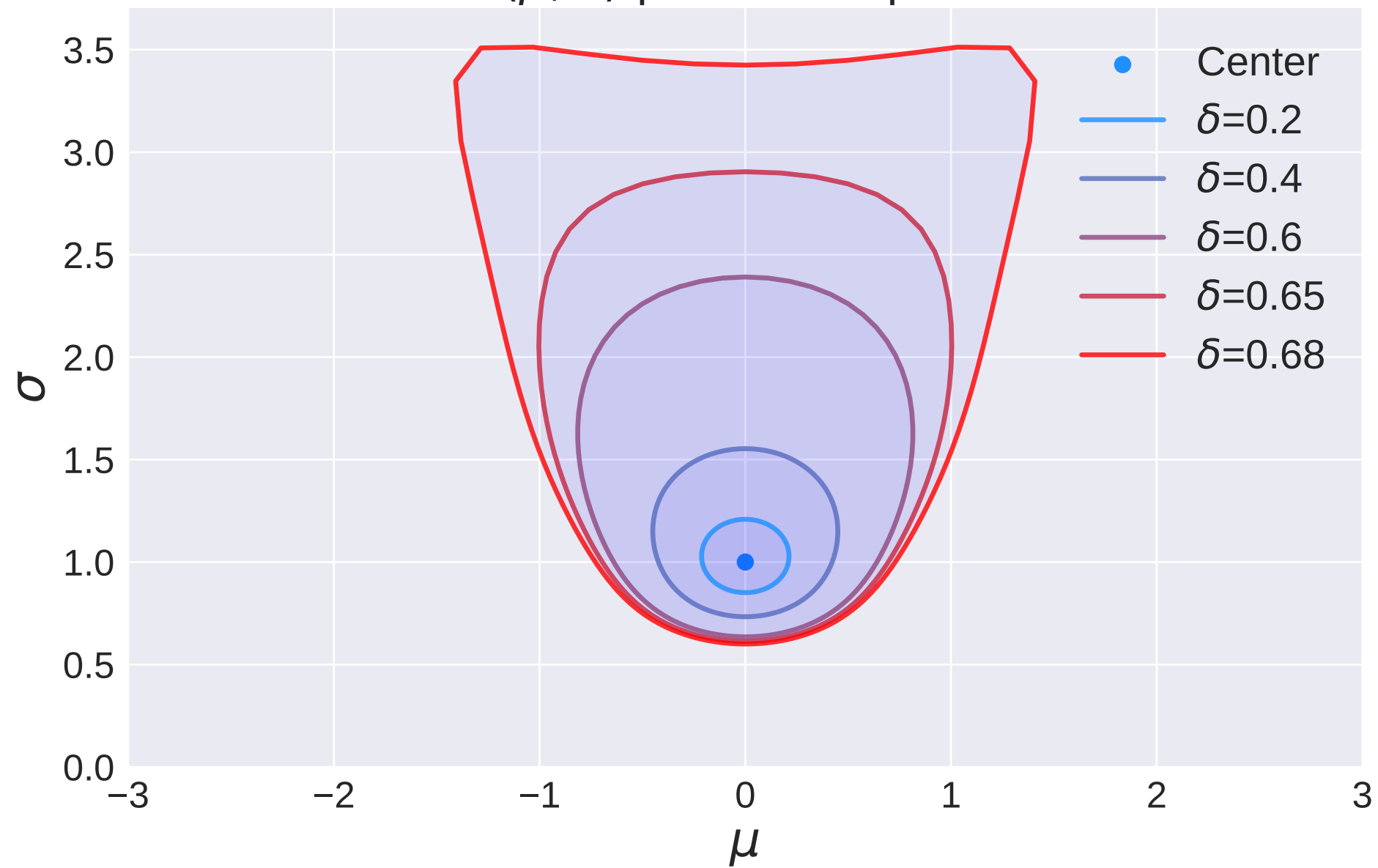
(\mu, \sigma) -parameter space
