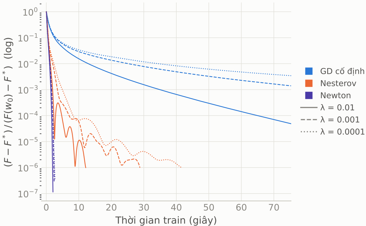
Ảnh hưởng của \lambda (số điều kiện)
