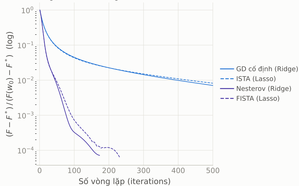
Ridge vs Lasso, cùng bước t = 2/L
