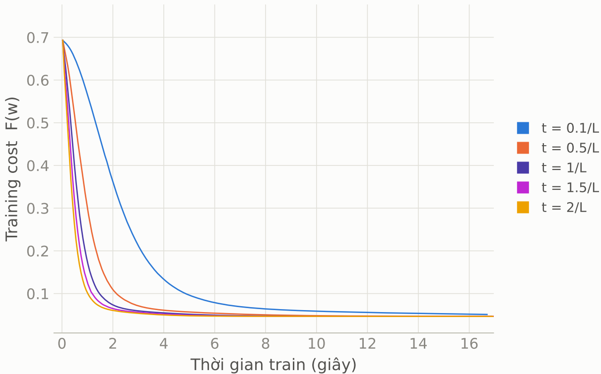
Proximal FISTA (Lasso)
