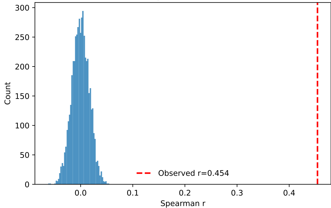
DINO V3 | Edge-value shuffle
