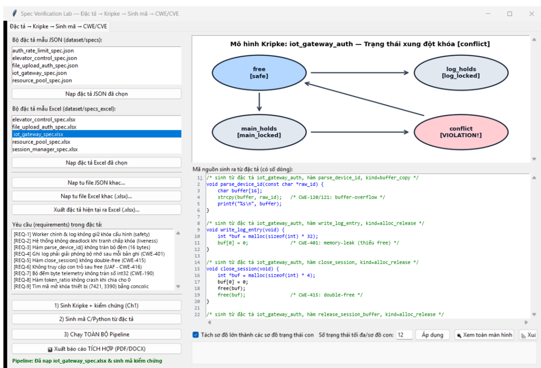
Hình: Minh chứng Ứng dụng: Giao diện SpecVerificationLab nạp và kiểm chứng thành công đặc tả SecureGate IoT Gateway
