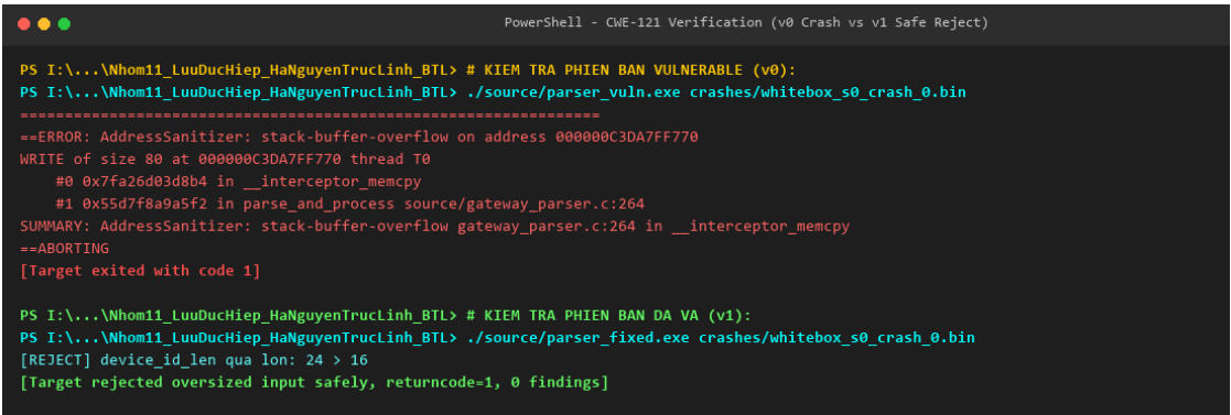
Hình: Minh chứng Thực nghiệm Terminal: So sánh trực diện v0 gây crash ASan và v1 từ chối an toàn
