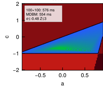
neutral DDE
