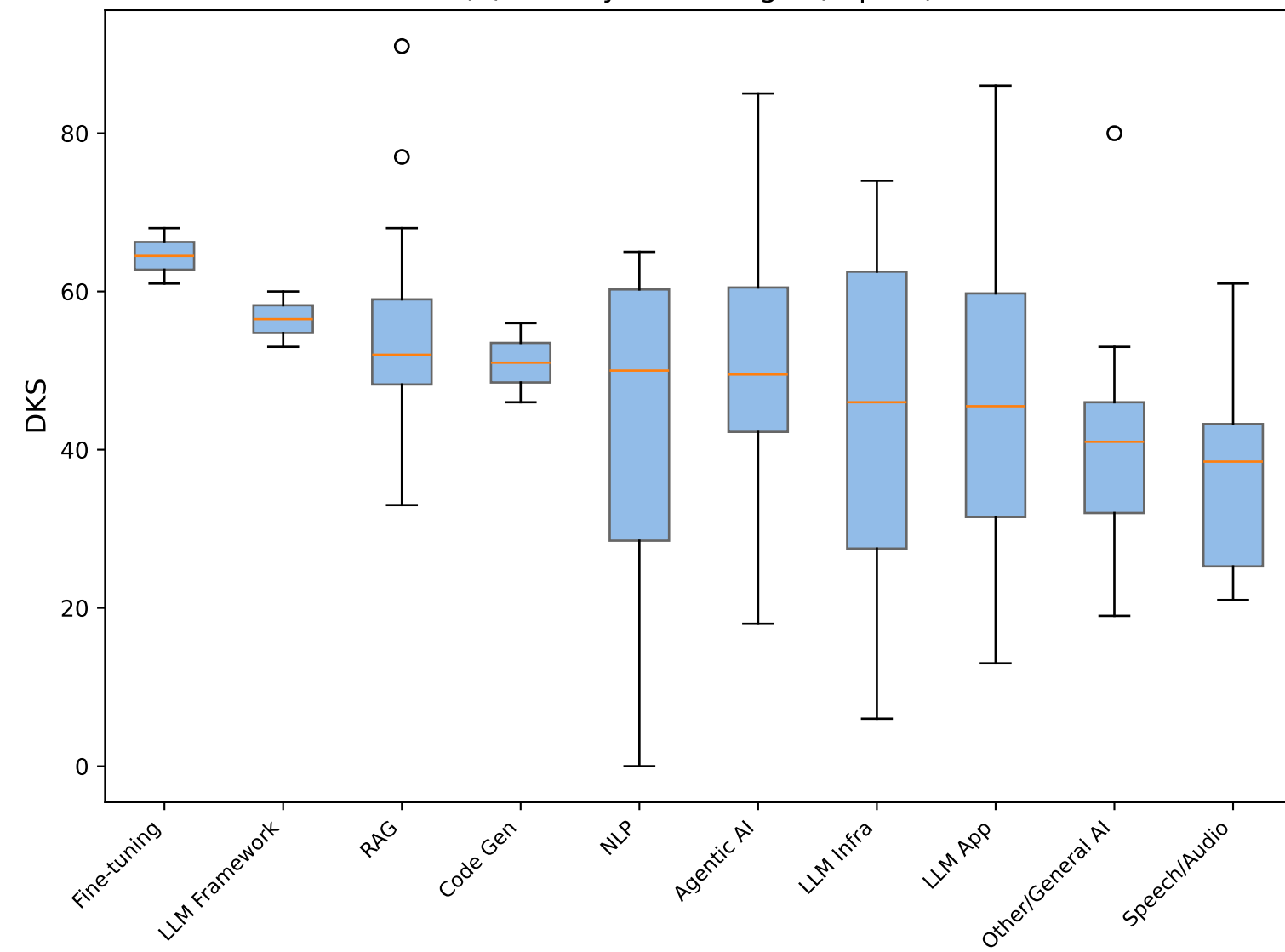
(d) DKS by AI Paradigm (Top 10)
