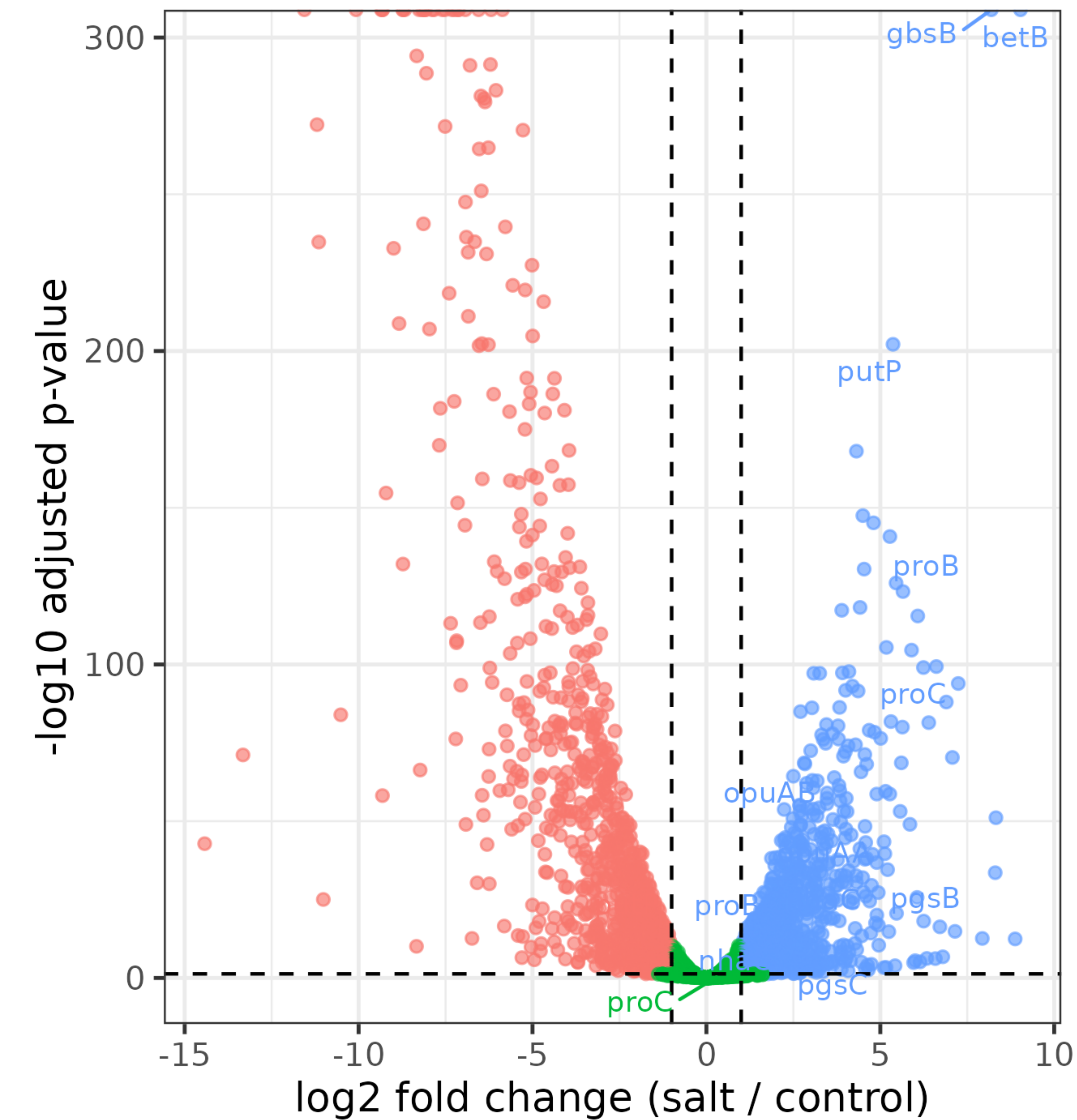
velezensis_control_vs_salt
