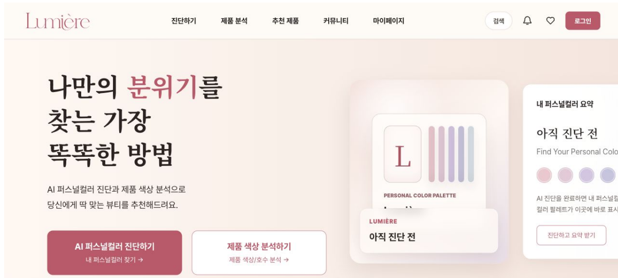
그림 1. 홈 화면
