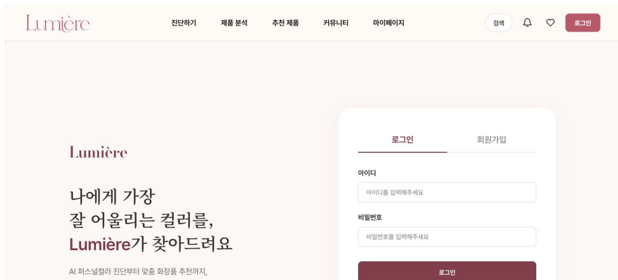
그림 2. 로그인/회원가입 화면
