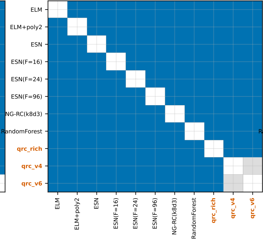
Lorenz-63
