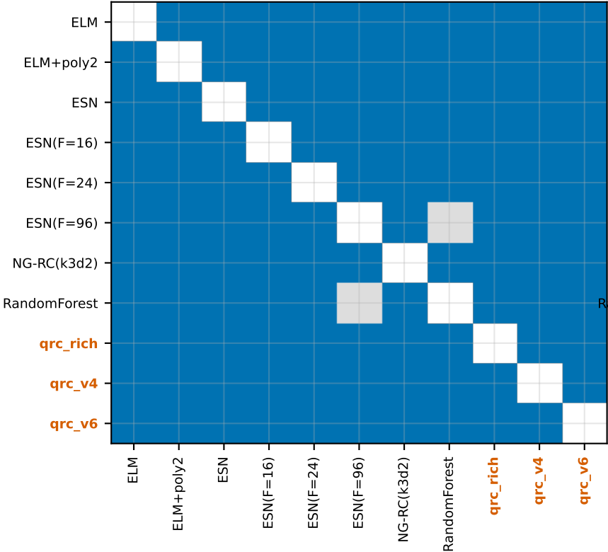
Hénon
