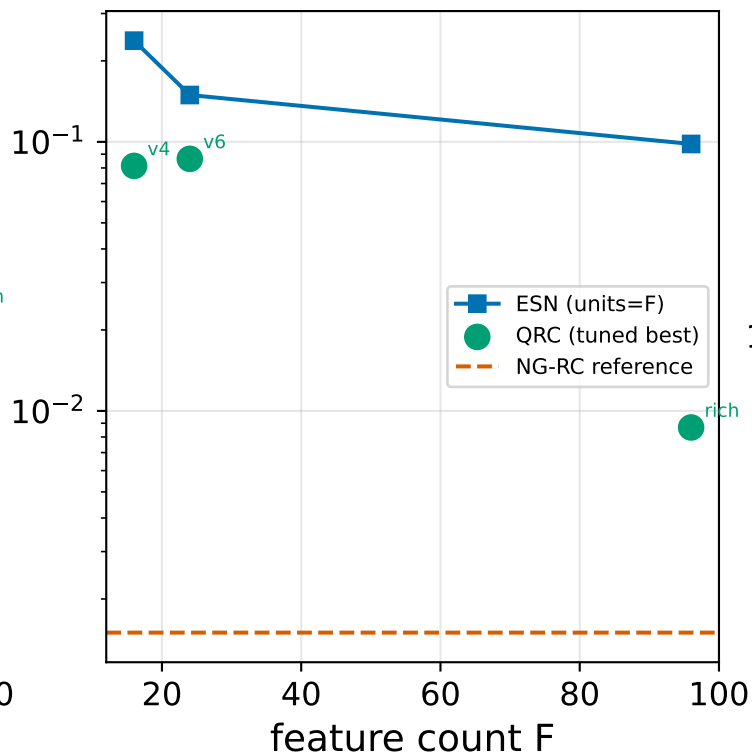
Lorenz-63
