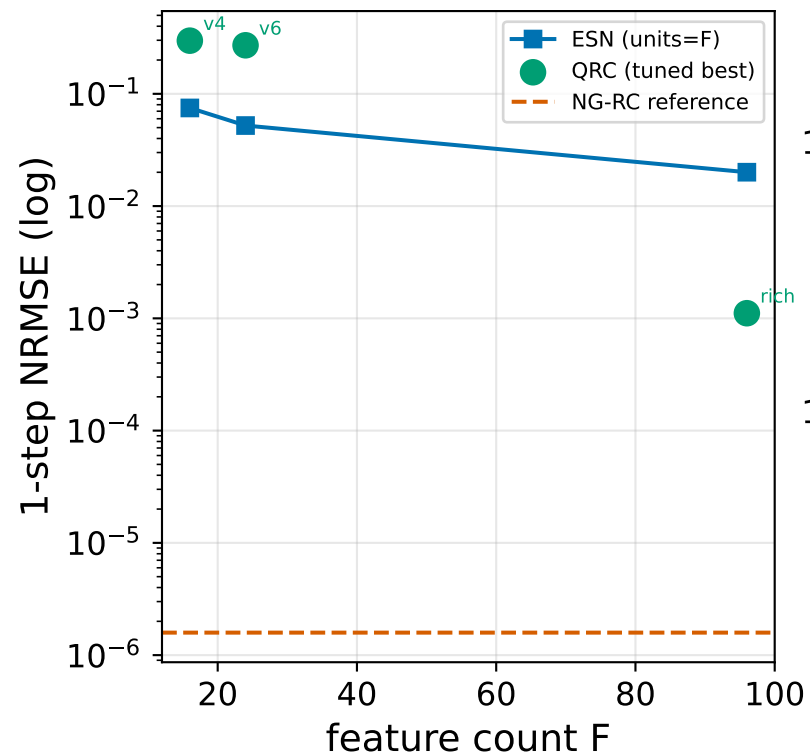
Hénon
