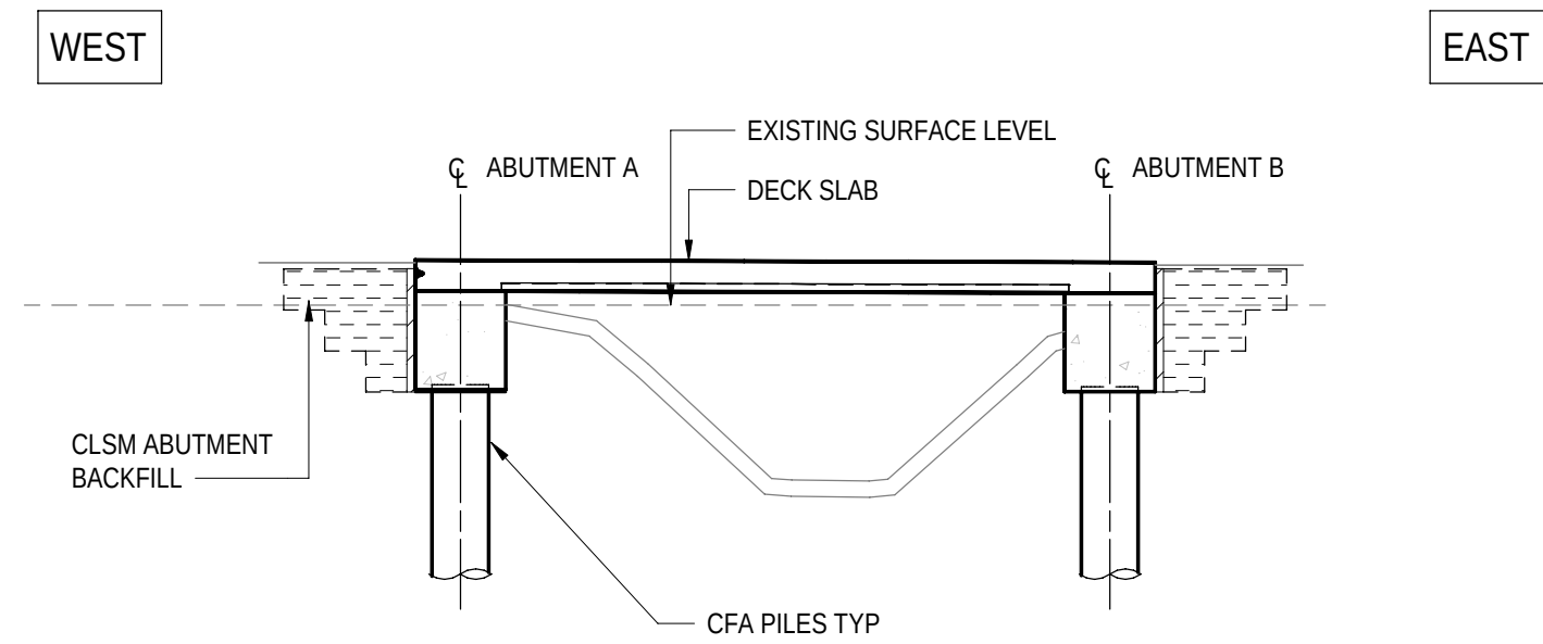
SECTION-STAGE A4
