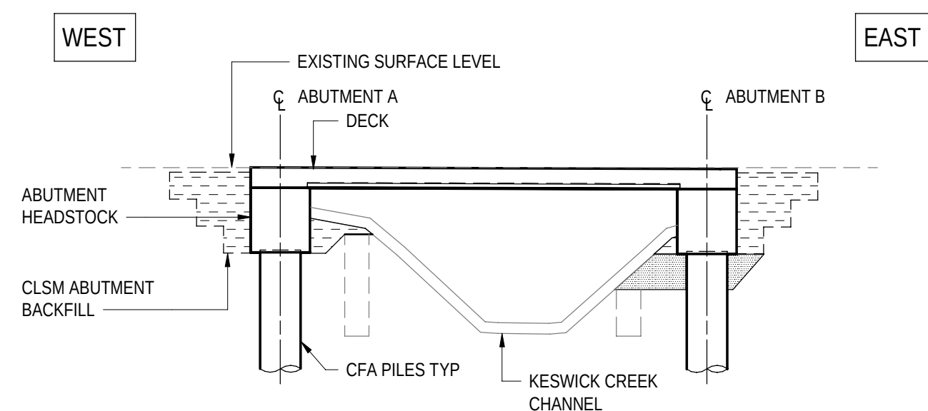
SECTION-STAGE B5
