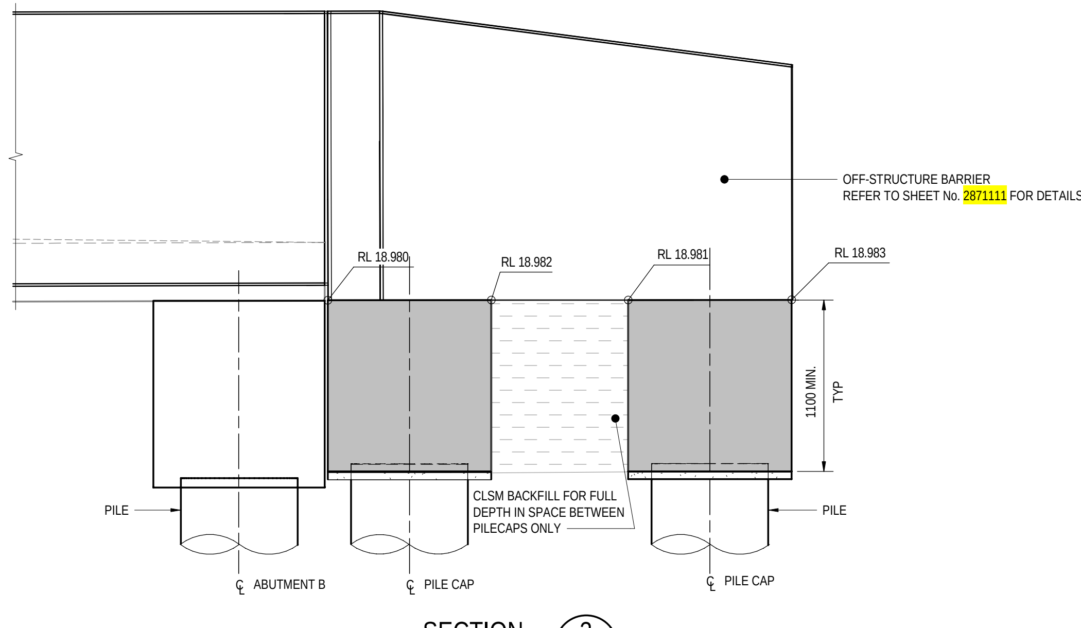
SECTION 3 SCALE 1 : 25
