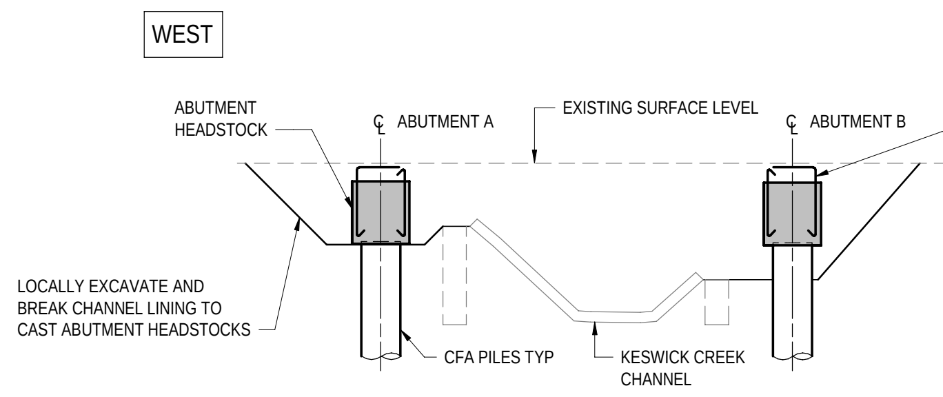
SECTION-STAGE B3
