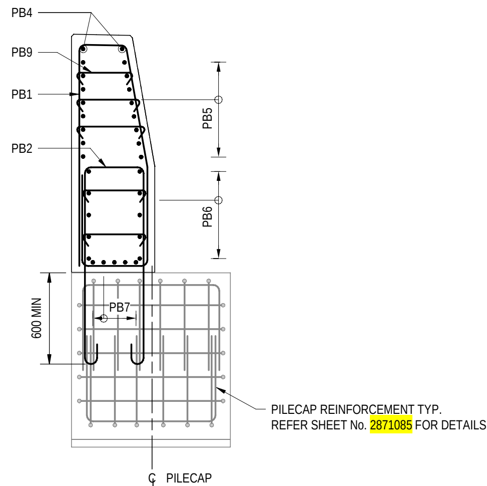
SECTION 1 SCALE 1 : 25
