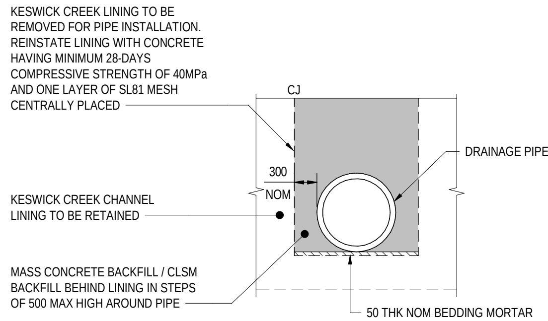
SECTION 4 SCALE 1 : 50 2871023
