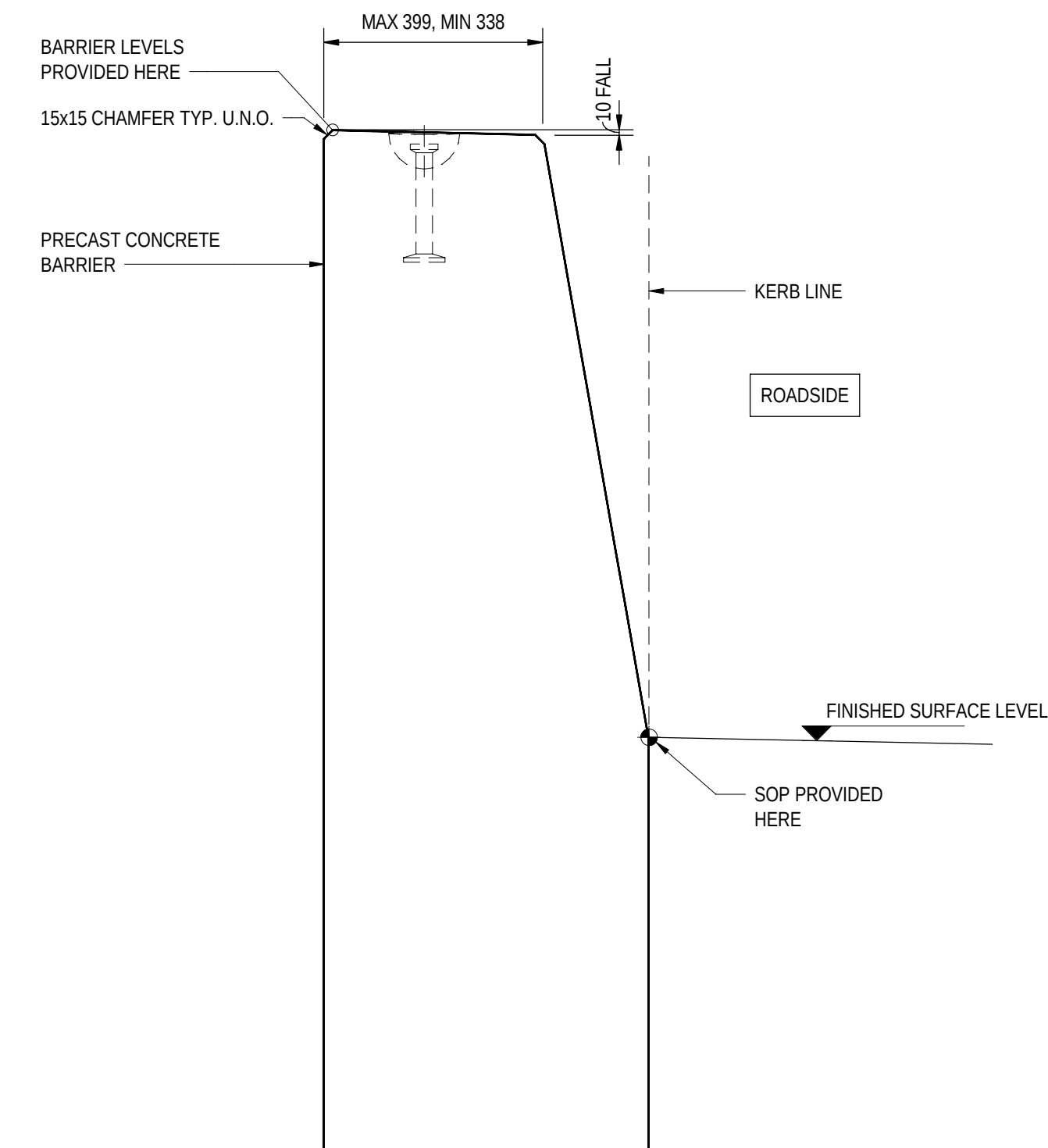
SECTION 1 SCALE 1 : 10
