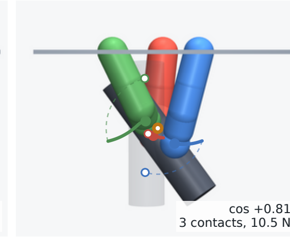
turn ramp 68 % (1.08 s)
