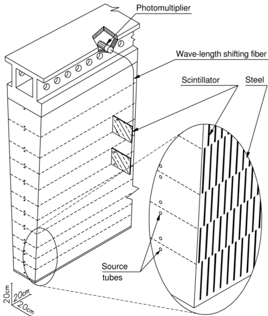
Tile Calorimeter wedge module
