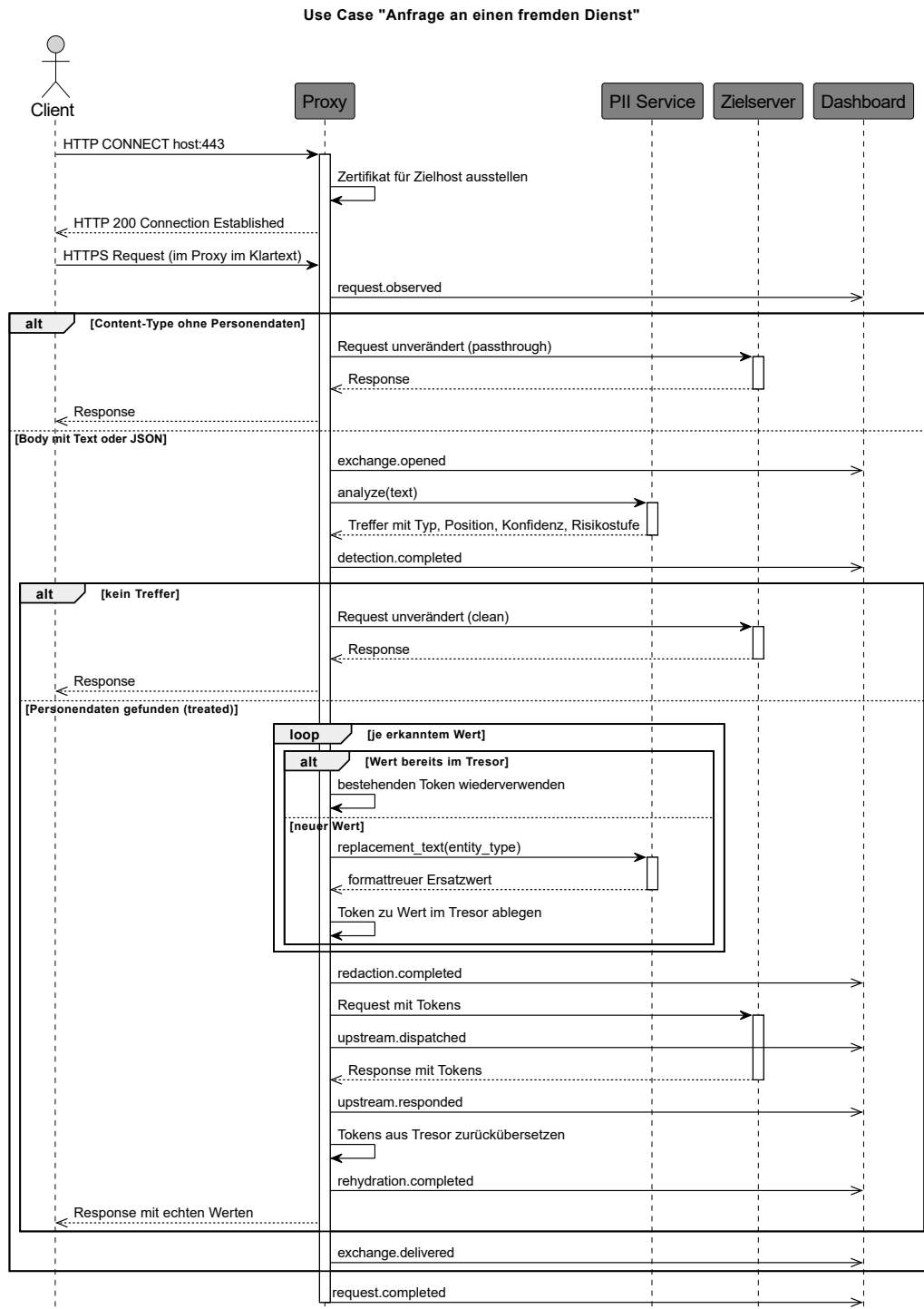
Abbildung 2: Das Software System zur Laufzeit.
