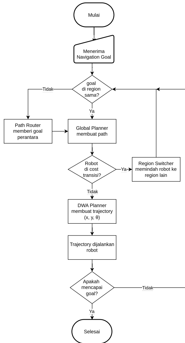
Gambar 3.9: Diagram alur navigasi
