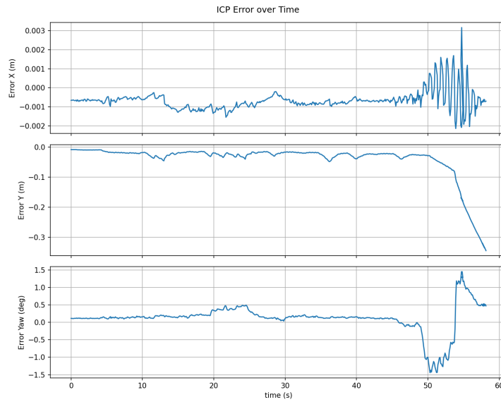
Gambar 4.1: Error ICP di Region A
