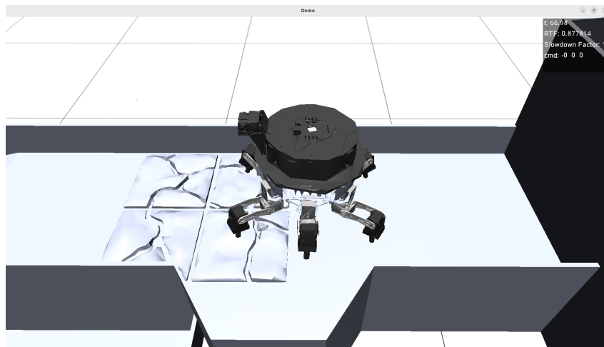
Gambar 3.17: Simulasi di Region A dengan rintangan lantai
