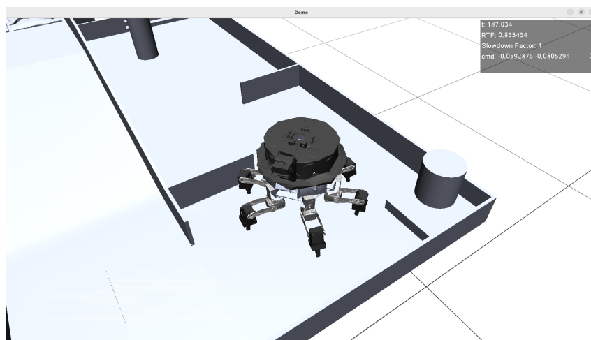
Gambar 3.18: Simulasi di Region C
