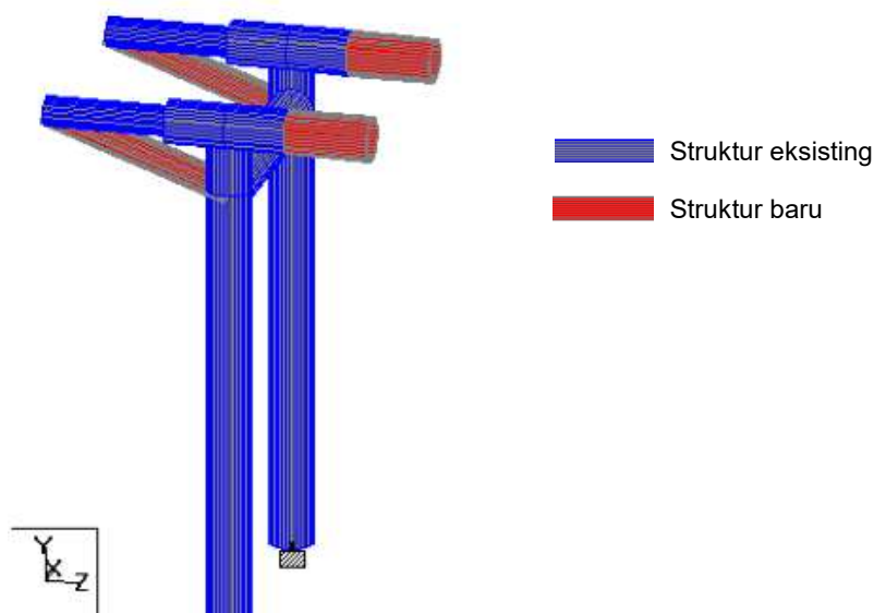
Pemodelan 3D di STAAD.Pro
