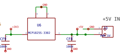
Alimentazione 5V -> 3,3V
