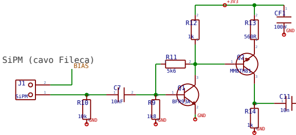
Amplificatore front-end SiPM
