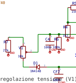
regolazione tensione (V1)
