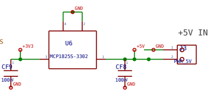
Alimentazione 5V -> 3,3V
