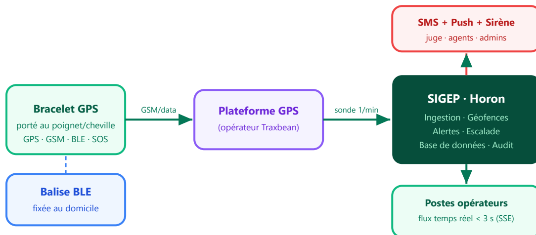
Figure 1 — Architecture générale : du bracelet au poste opérateur, chaque position transite par la sonde (1/minute), est confrontée aux géofences, et déclenche alertes et notifications le cas échéant.
