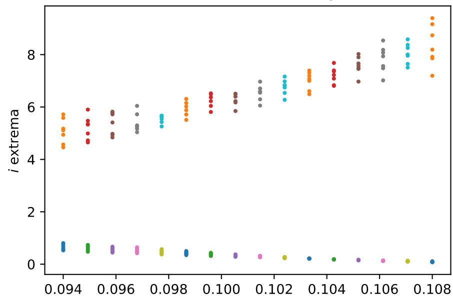
(d) infection rate \lambda
