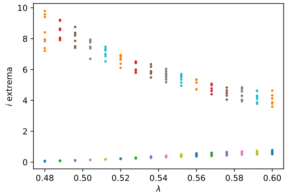
(d) infection rate \lambda
