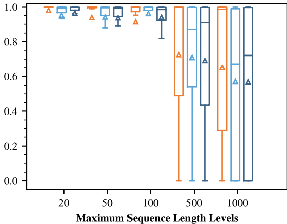
F1 Score for Failure Class
