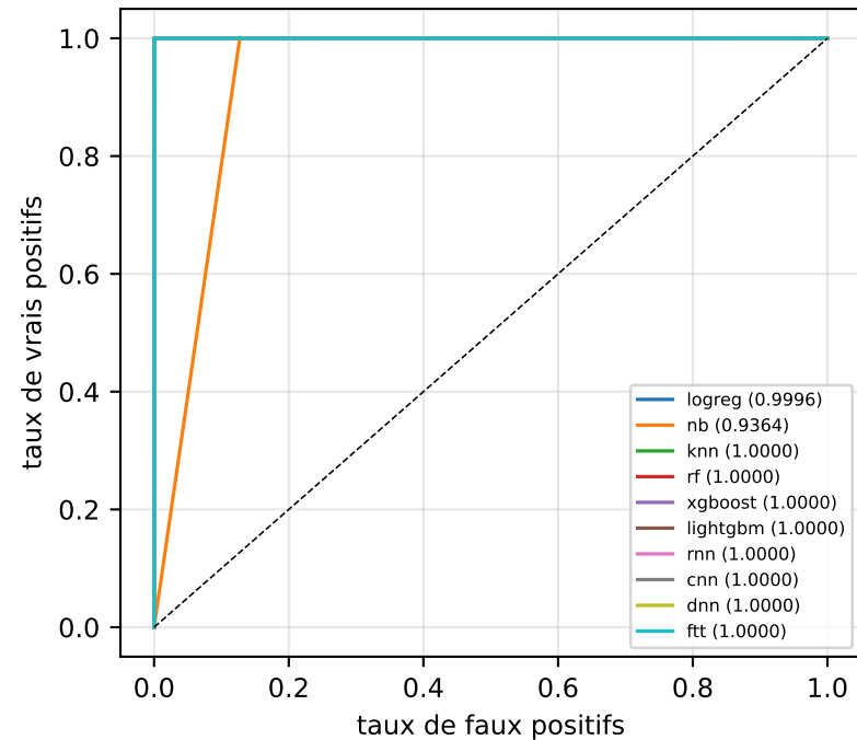
ROC — benin vs attaque
