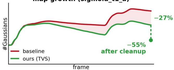
(d) map growth (sigmoid_t1_a)
