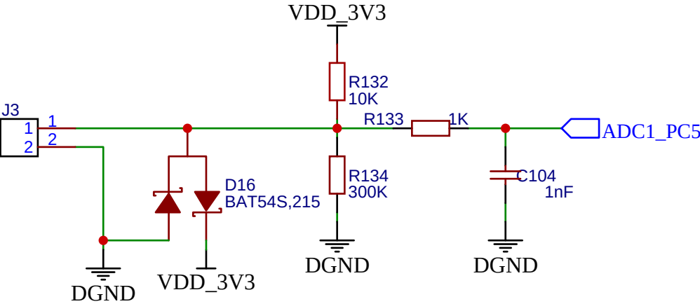
接温控探头 (NTC)
