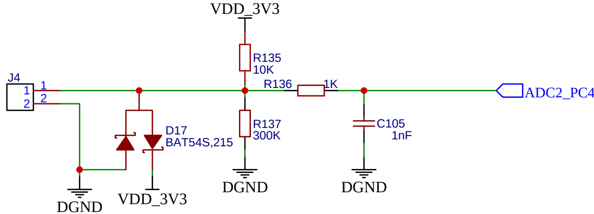
接温控探头 (NTC)
