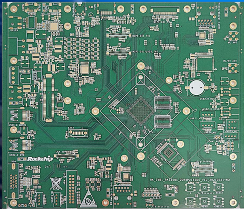
十四层三阶HDI板
