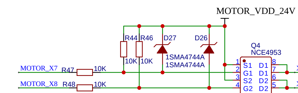
X(行)驱动电路
