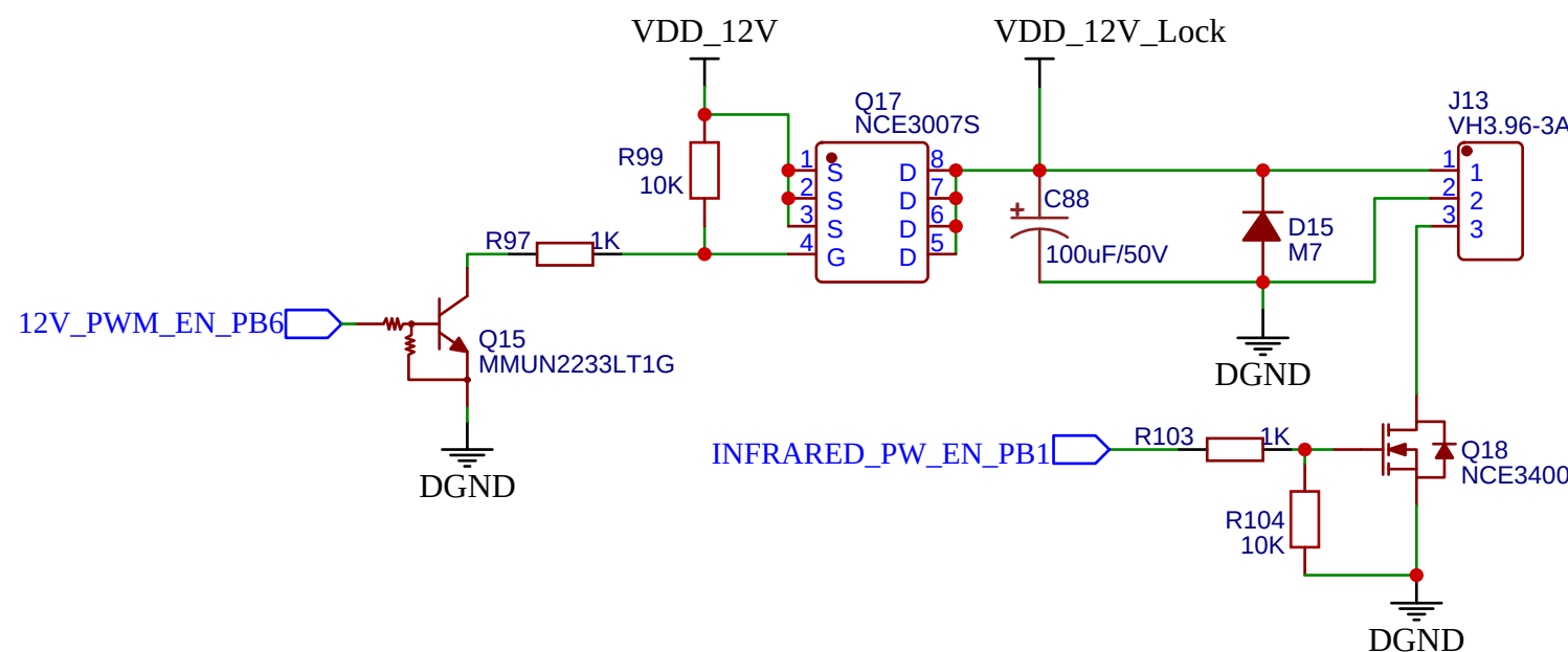
门锁电源及控制
