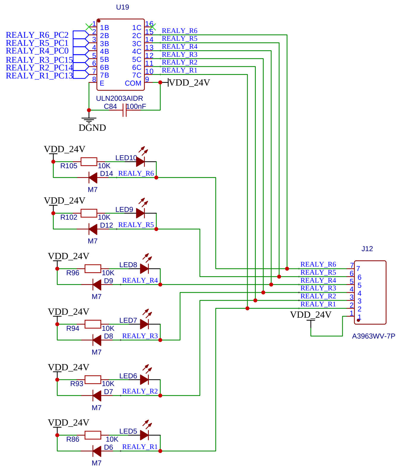
继电器控制电路
