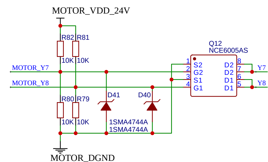
Y(列)驱动电路
