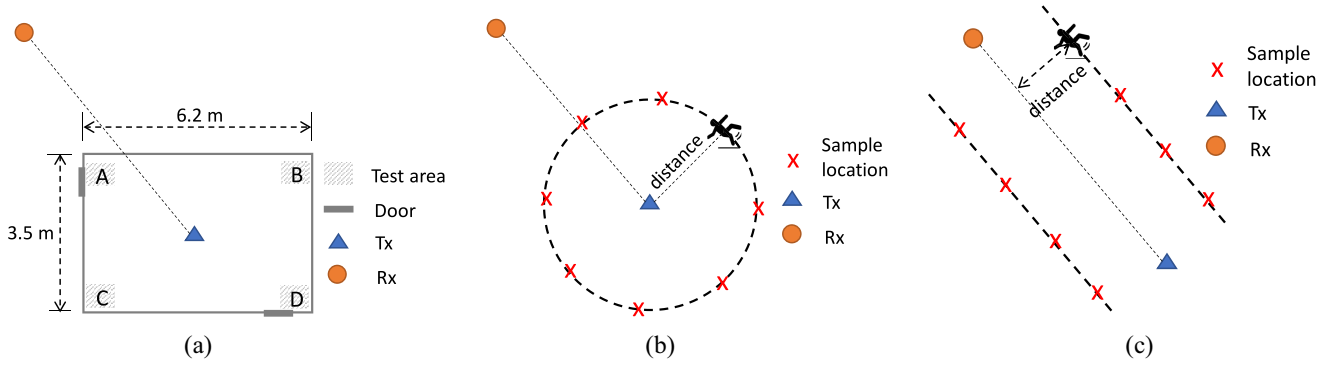
Fig. 12. Settings for analyzing coverage. (a) Setting 1: NLOS scenario. (b) Setting 2: LOS scenario. (c) Setting 3: LOS scenario.
