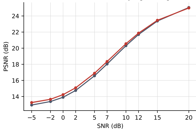
(d) k = 4 PSNR under Rayleigh fading
