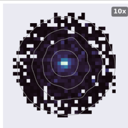
DiffuRec
