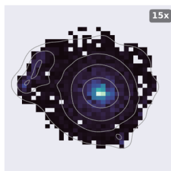
SASRec
