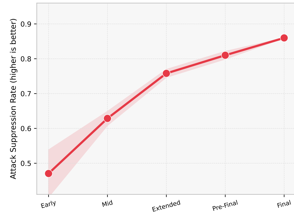
A2C
