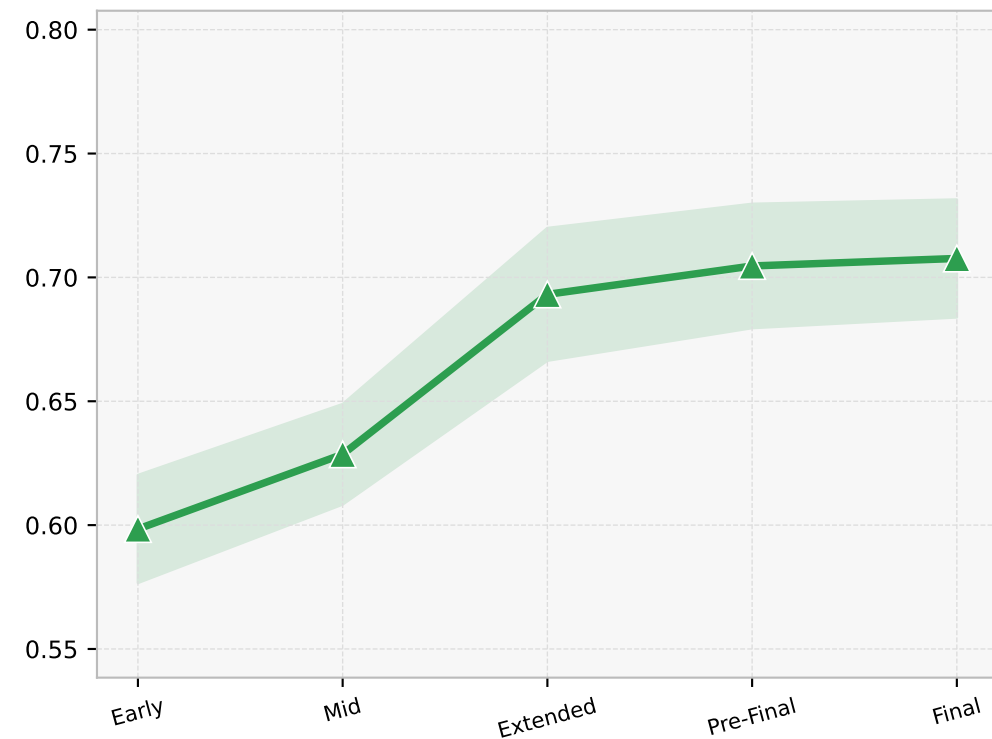
Baseline
