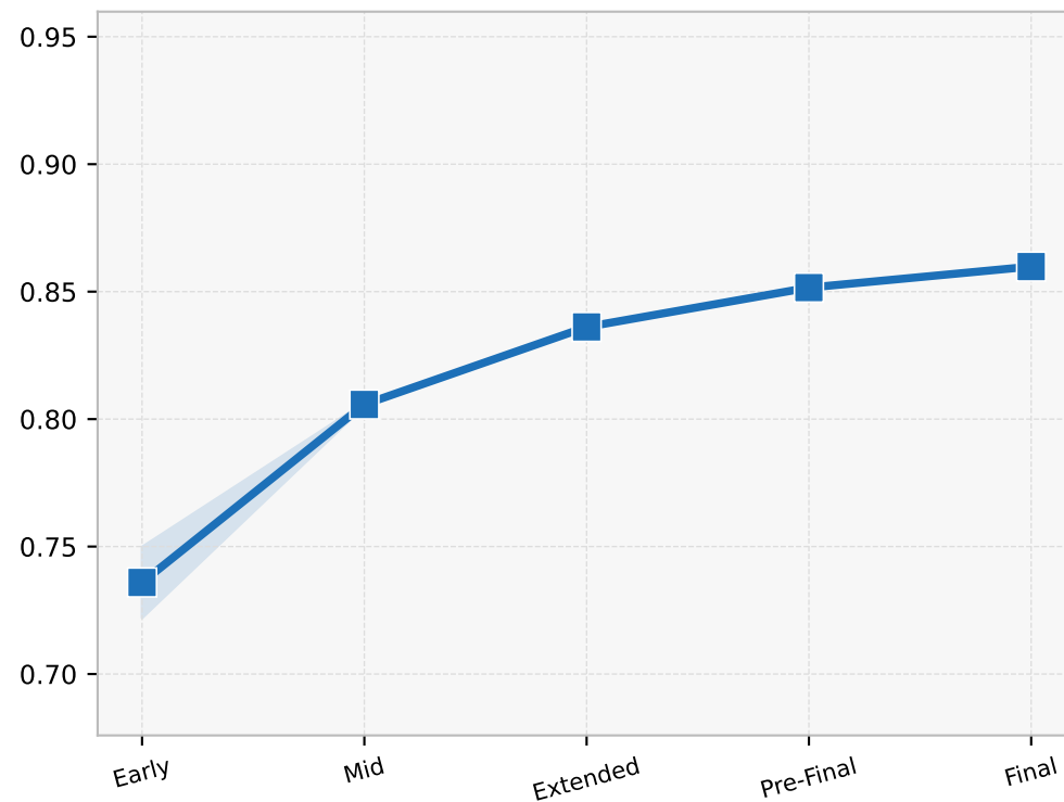
TD3
