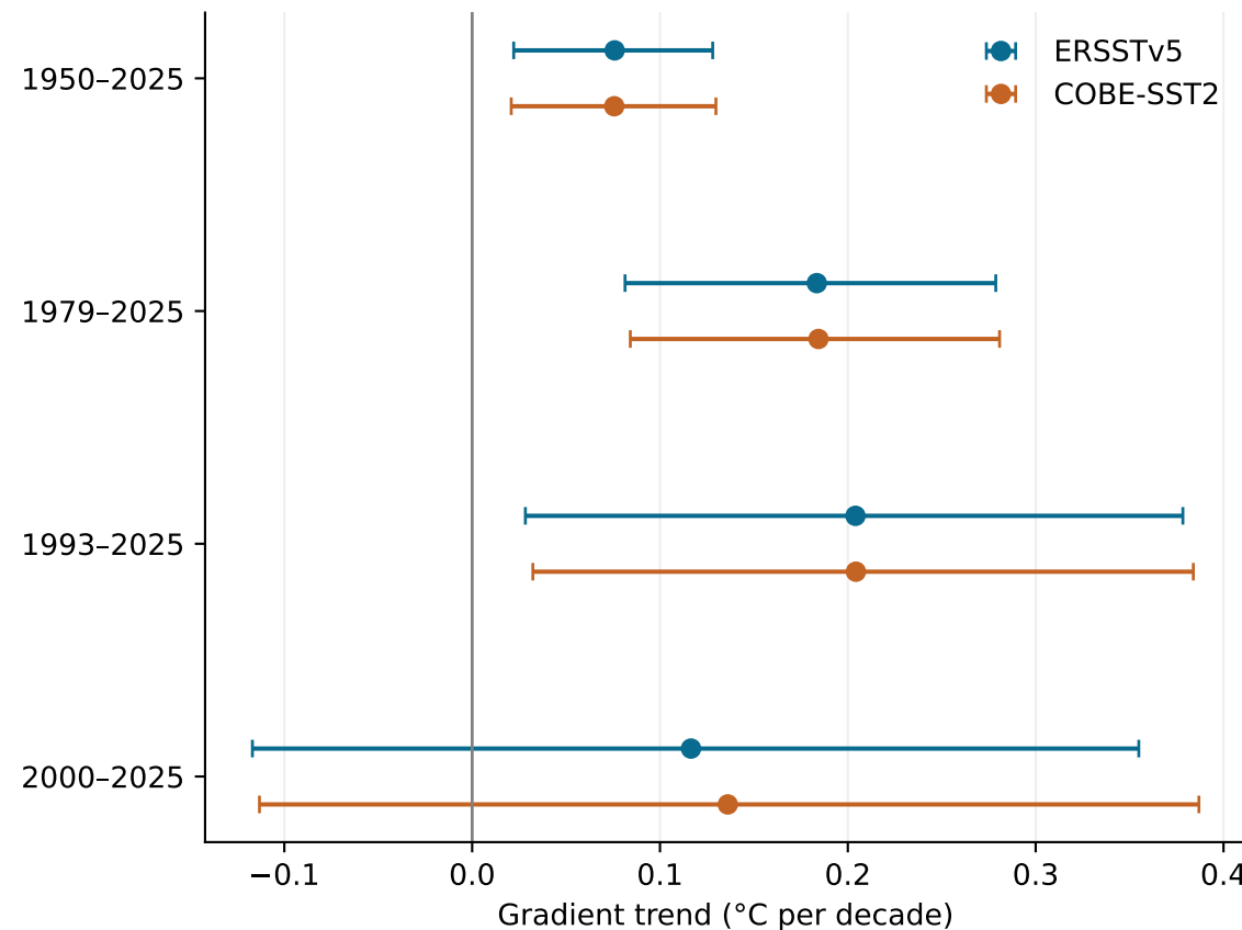
Latitude: 3°S-3°N
