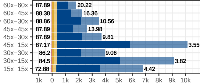
COLO829
