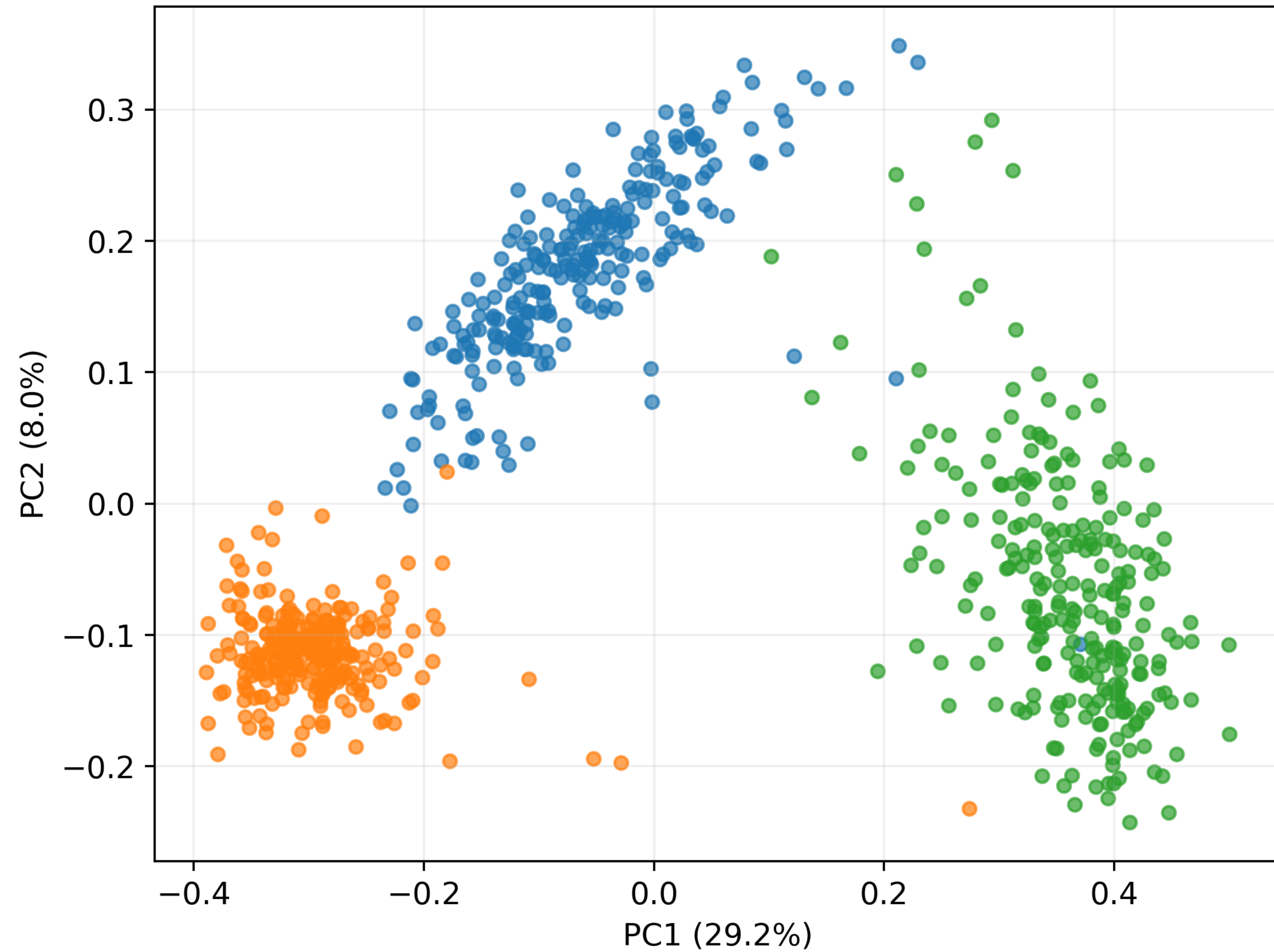
paligemma2 pixelprose, layer 20
