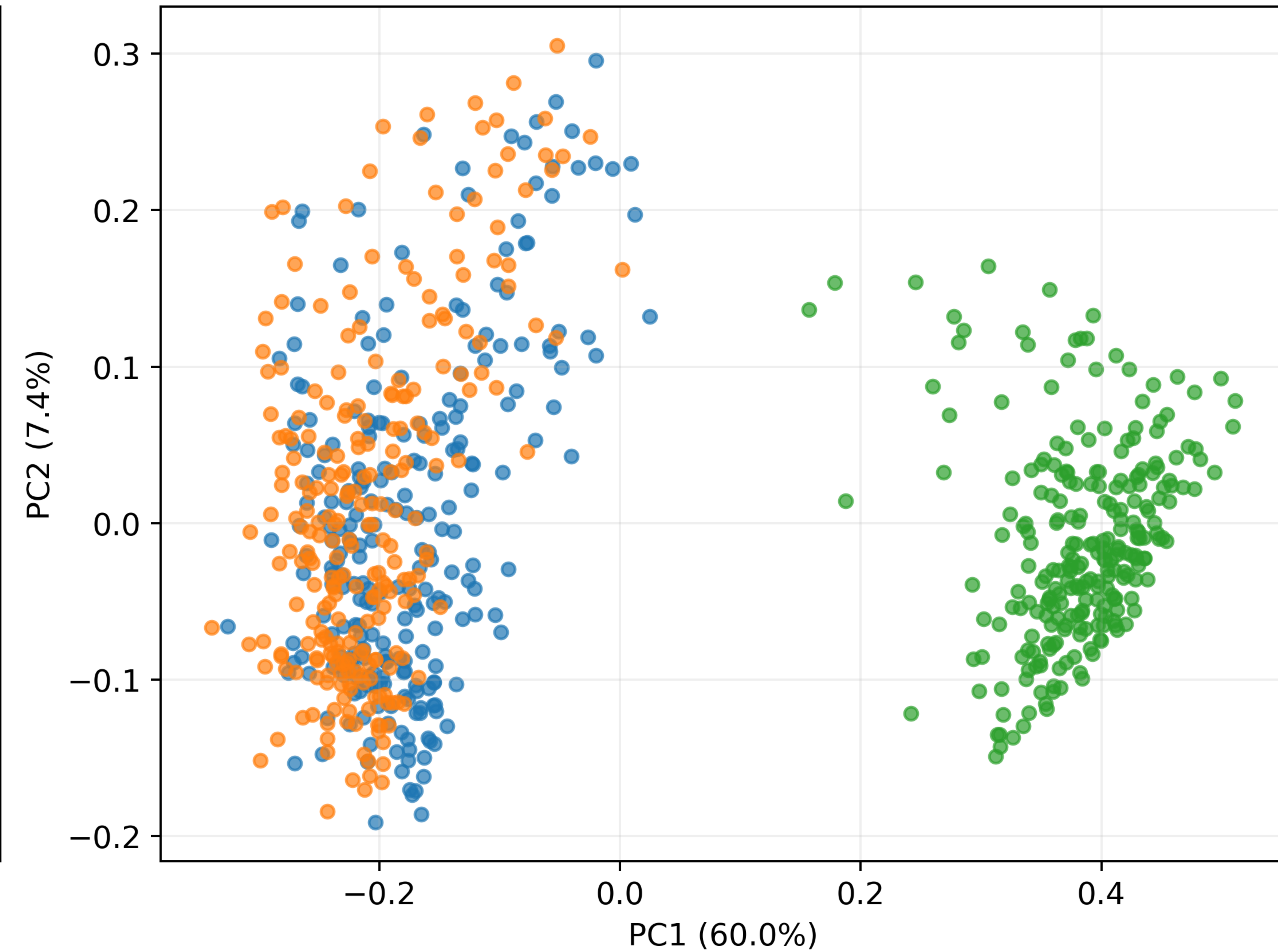
smolvlm pixelprose, layer 24
