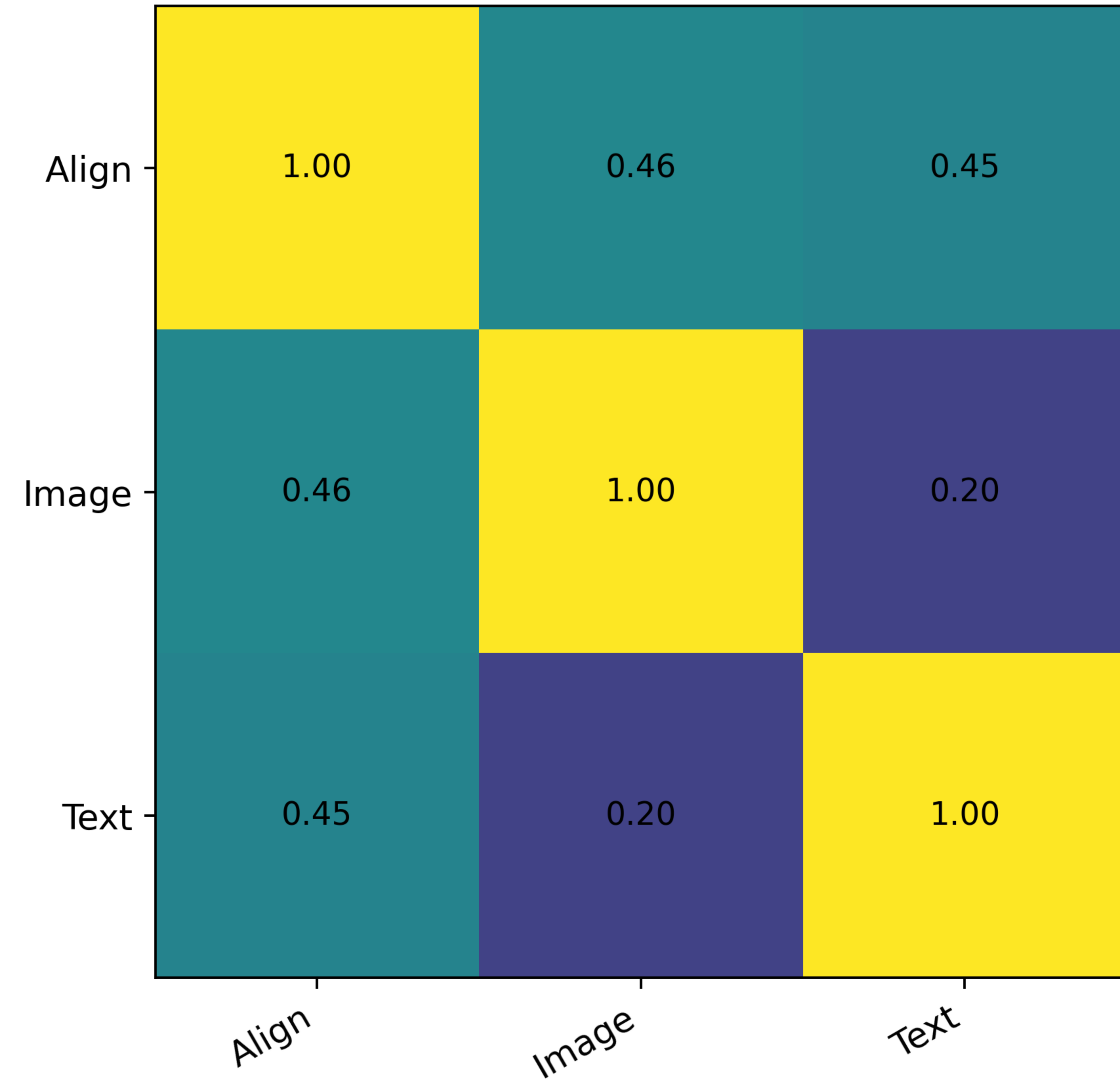
paligemma2 pixelprose, layer 20
