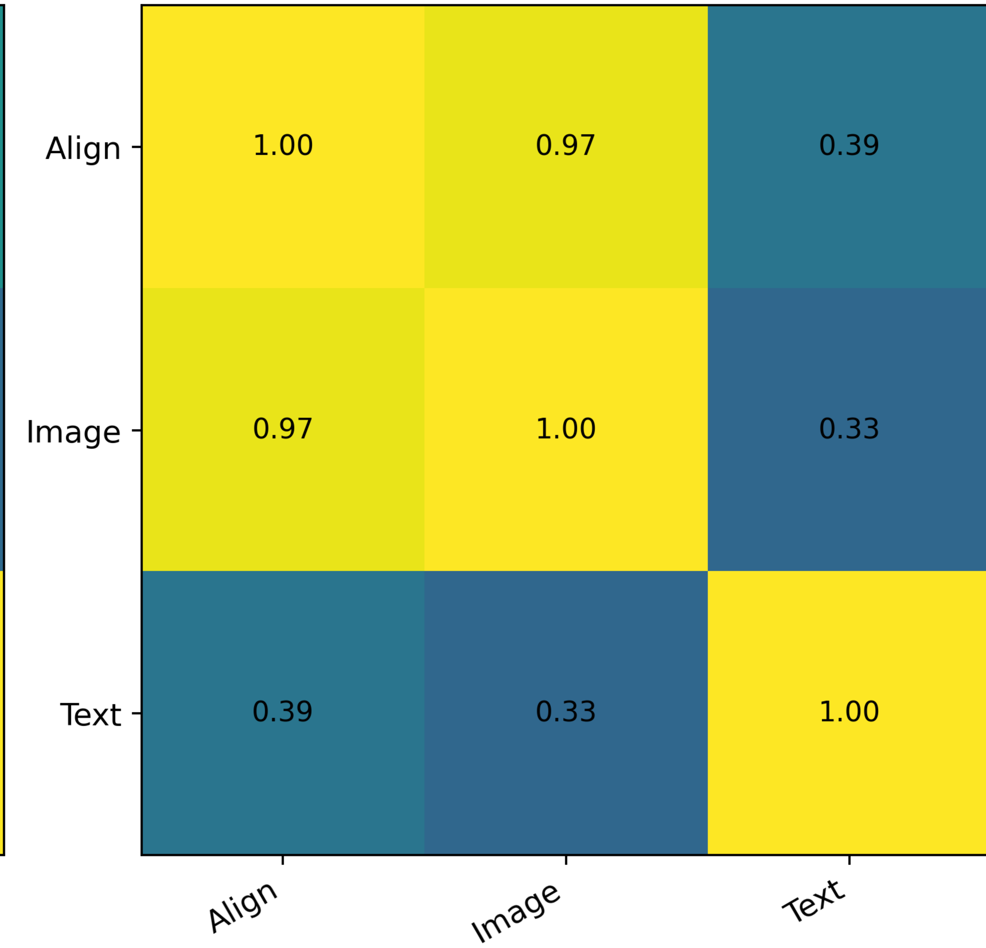
smolvlm pixelprose, layer 24
