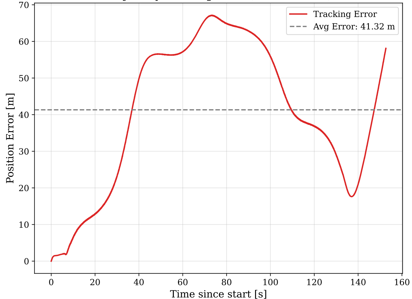
Trajectory Tracking Error (Max: 67.13 m)
