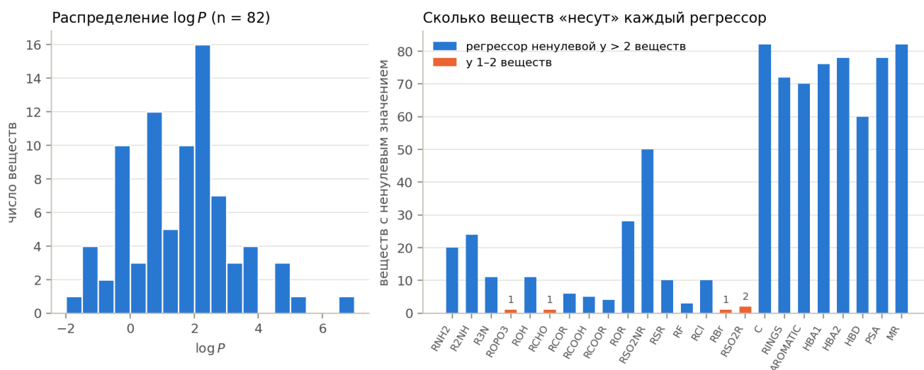
Рисунок 1. Слева — распределение \log P . Справа — у скольких веществ регрессор отличен от нуля. ROPO3, RCHO и RBr встречаются по одному разу, RSO2R — дважды.
