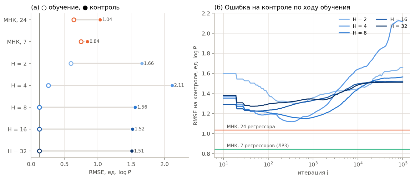
Рисунок 5. (а) Ошибка на обучении ( \circ ) и на контроле ( \bullet ). (б) Ошибка на контроле по ходу обучения перцептрона. Горизонтальные линии — линейные модели ЛРЗ.
