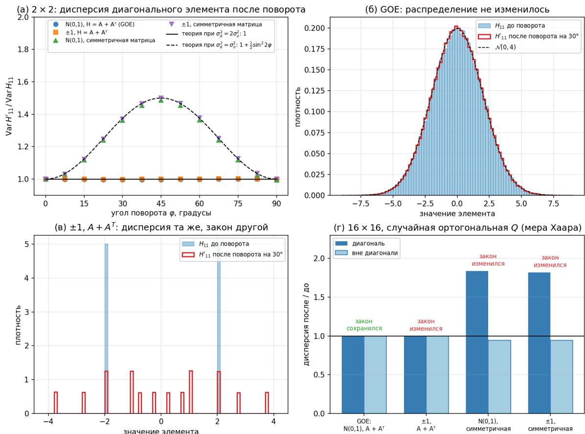
Рисунок 1. (а) Матрицы 2×2, поворот на угол \varphi : дисперсия H'_{11} относительно исходной. Точки — моделирование, линии — формула \text{Var} H'_{11} = \sigma_d^2(1 - \frac{1}{2}\sin^2 2\varphi) + \sigma_o^2 \sin^2 2\varphi . (б) GOE: распределение H_{11} до и после поворота на 30°. (в) То же для A + A^T с A из \pm 1 . (г) Матрицы 16×16 и случайная Q по мере Хаара.
