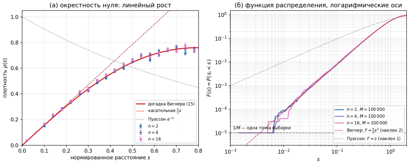
Рисунок 4. (а) Начало гистограмм крупным планом, с погрешностями. (б) Эмпирическая функция распределения в логарифмических осях.
