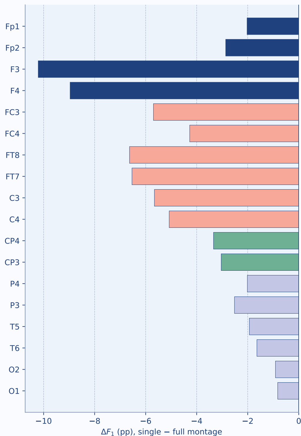
Cao2018
